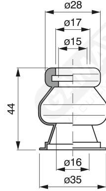
Art. VSS 35/1
