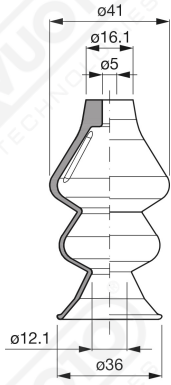
Art. VSS 34/2
