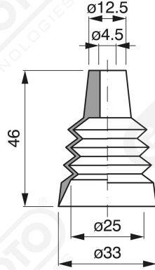
Art. VSS 33/3
