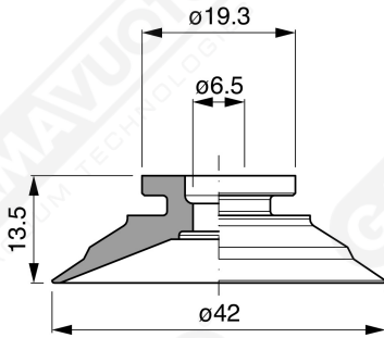
Art. CF 40 15
