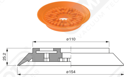
Art. AF 150 45
